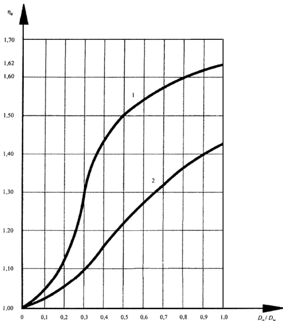
График для определения коэффициента несущей способности тройников
