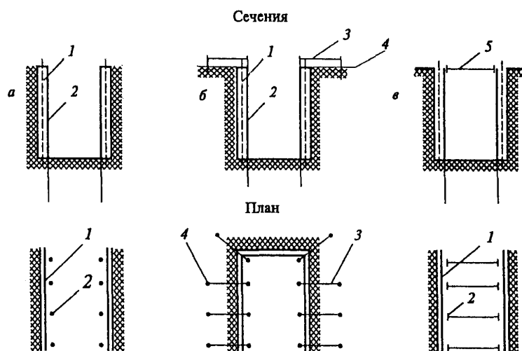
Рис. 5.3. Схемы консольных креплений: а - безраспорное; б - анкерное; в - консольно-распорное; 1 - затяжки; 2 - сваи; 3 - растяжки; 4 - анкер; 5 - распорки
