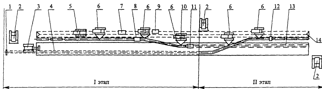
Рис. 3.1. Технологическая схема капитального ремонта трубопроводов с заменой труб путем укладки в совмещенную траншею:
