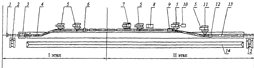
Рис. 3.3. Технологическая схема капитального ремонта трубопроводов с заменой труб путем укладки на существующее ложе:
