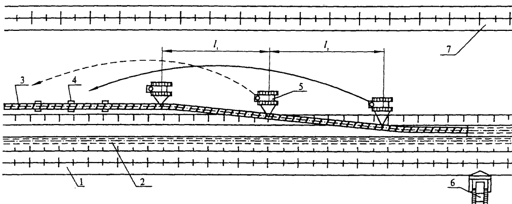
Рис. 6.2. Расстановка машин и механизмов при раздельном способе изоляционно-укладочных работ:
