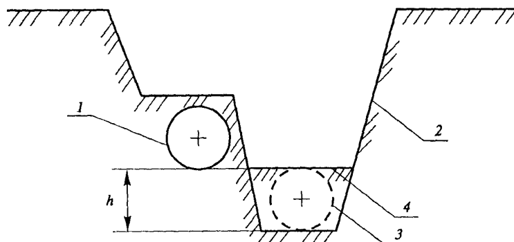
Рис. 5.2. Профиль траншеи при ремонте с заменой труб путем укладки в совмещенную траншею ниже существующего трубопровода: 1 - заменяемый участок трубопровода; 2 - траншея; 3 - вновь прокладываемый участок трубопровода; 4 - перемычка; h - величина заглубления
