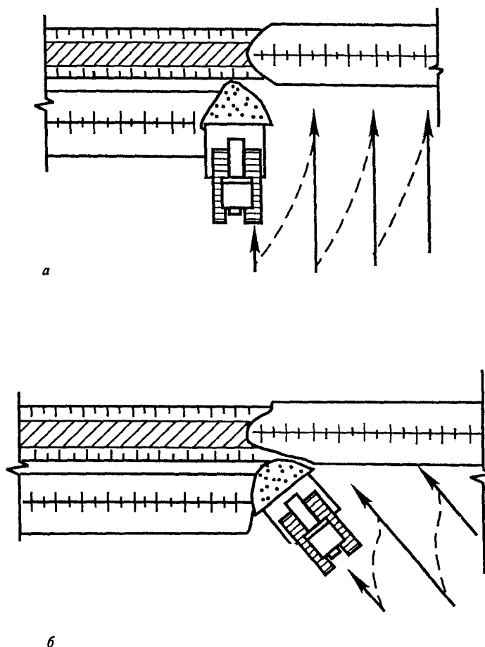
Рис. 5.7. Схемы производства работ по засыпке уложенного трубопровода бульдозером: а - прямолинейными проходами; б - косопоперечными параллельными проходами
