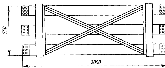
Рис. 5.4. Неинвентарные крепления траншеи: а - простейшее; б - анкерное;
