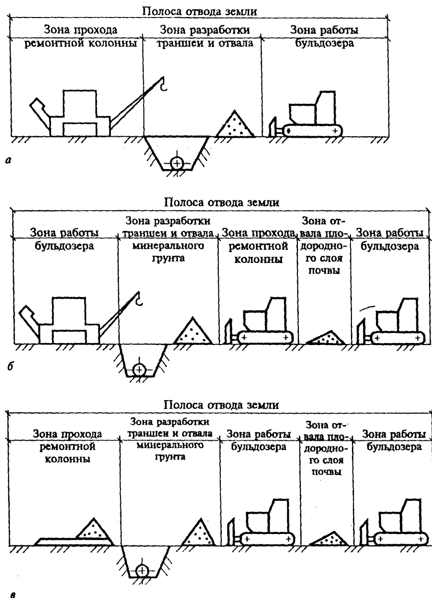
Рис. 5.6. Варианты размещения отвалов минерального и плодородного грунта относительно оси трубопровода: а - без рекультивации земли; б, в - с рекультивацией земли
