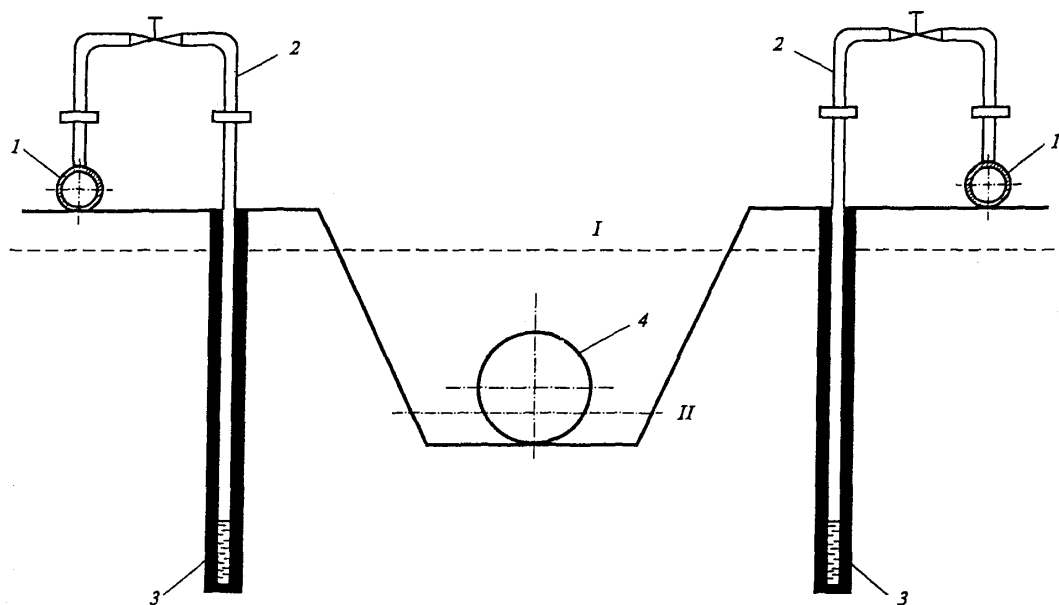
Рис. 5.5. Схема искусственного водопонижения при двух рядах иглофильтров:
