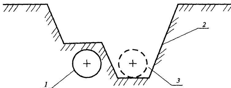
Рис. 5.1. Профиль траншеи при ремонте с заменой труб путем укладки в совмещенную траншею: 1 - заменяемый участок трубопровода; 2 - траншея; 3 - вновь прокладываемый участок трубопровода
