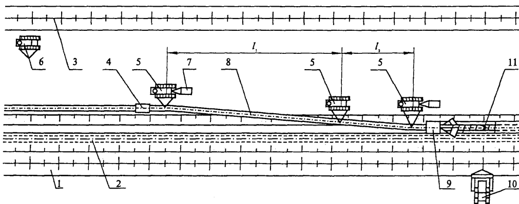
Рис. 6.1. Расстановка машин и механизмов при совмещенном способе изоляционно-укладочных работ:
