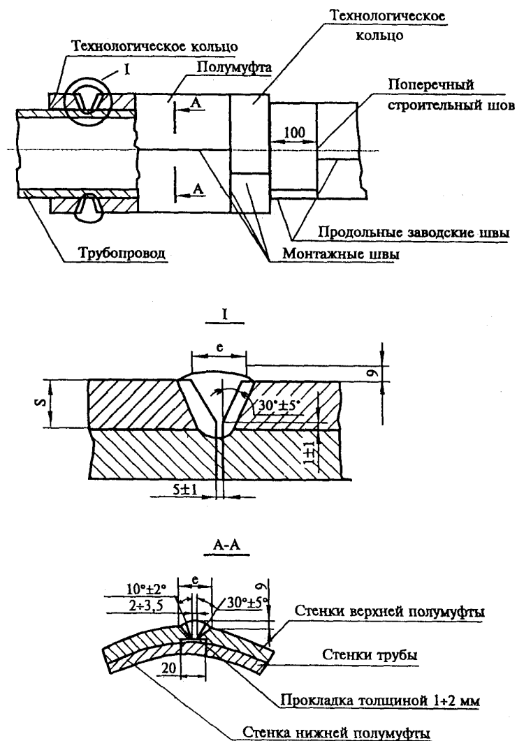
Рис. 8.1. Схема монтажа и сборки муфты с технологическими кольцами
